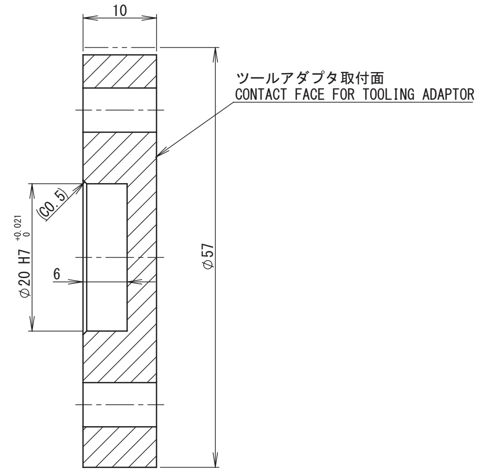
断面図 A-A SECTION A-A
